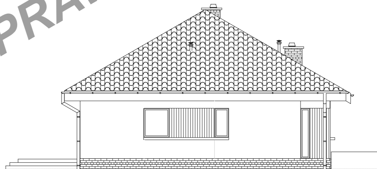
elwacja boczna 2
